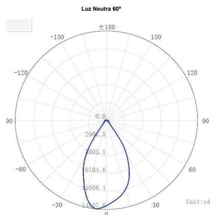
Curva de Distribución Luminosa
